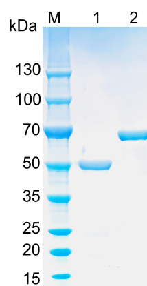
Recombinant Arabidopsis thaliana ATSOS2 SDS-PAGE
