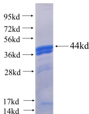
Recombinant human STRBP SDS-PAGE
