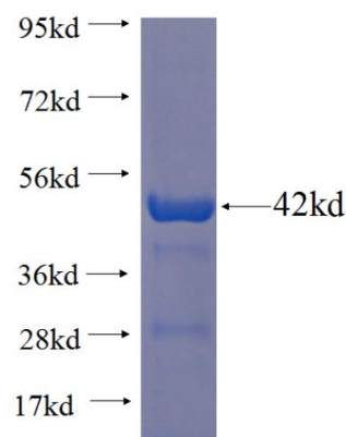
Recombinant Arabidopsis thaliana CeQORH SDS-PAGE
