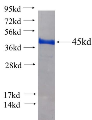
Recombinant human HMG20A SDS-PAGE
