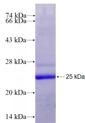
Recombinant Human MYCBP2 SDS-PAGE
