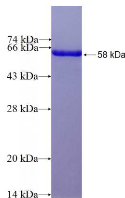
Recombinant Human BNC1 SDS-PAGE
