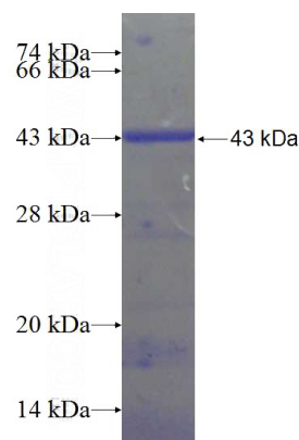
Recombinant Human POU2F2 SDS-PAGE
