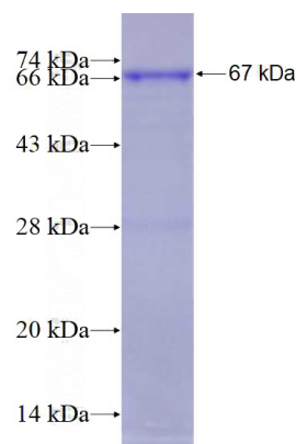
Recombinant Human FER SDS-PAGE
