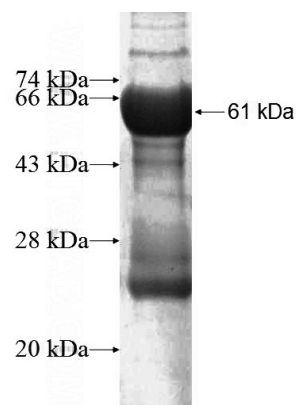
Recombinant Human RALGPS1 SDS-PAGE
