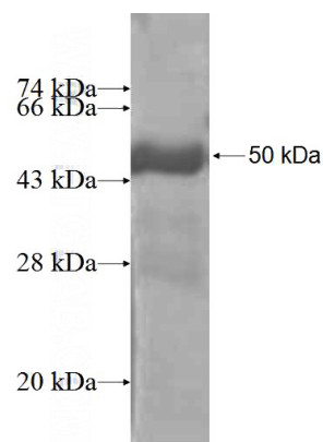
Recombinant Human DUSP19 SDS-PAGE
