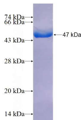
Recombinant Human RARS SDS-PAGE
