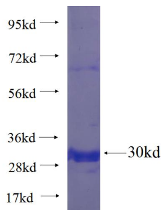
Recombinant human TRPC5 SDS-PAGE
