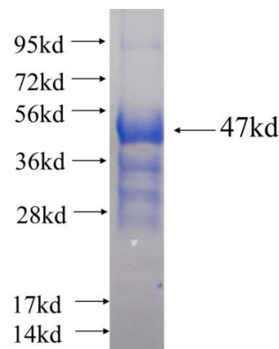
Recombinant human NANOS3 SDS-PAGE
