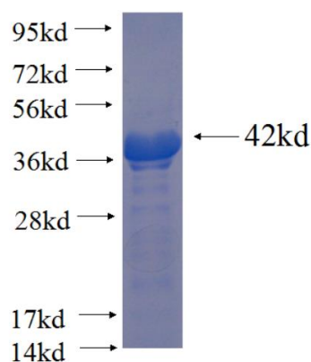
Recombinant human KIAA0586 SDS-PAGE
