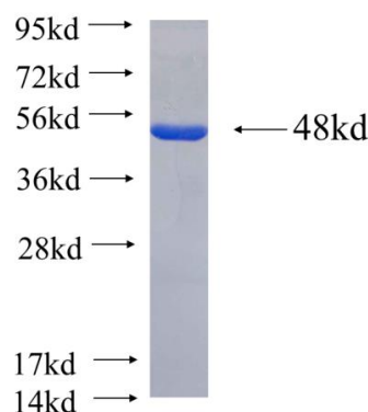
Recombinant Arabidopsis thaliana ATDEF2 SDS-PAGE
