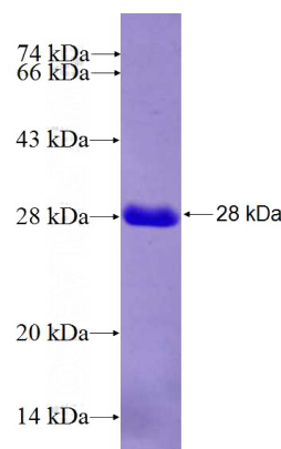
Recombinant Human ELF4 SDS-PAGE
