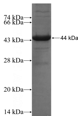
Recombinant Human RORC SDS-PAGE
