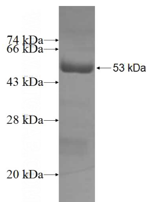
Recombinant Human TNNT1 SDS-PAGE
