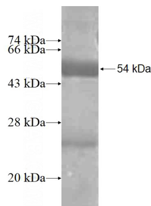
Recombinant Human GIMAP2 SDS-PAGE
