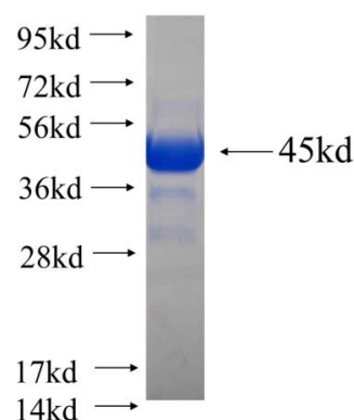
Recombinant human CIAPIN1 SDS-PAGE
