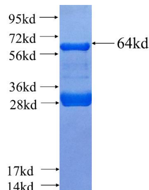
Recombinant human AFG3L2 SDS-PAGE
